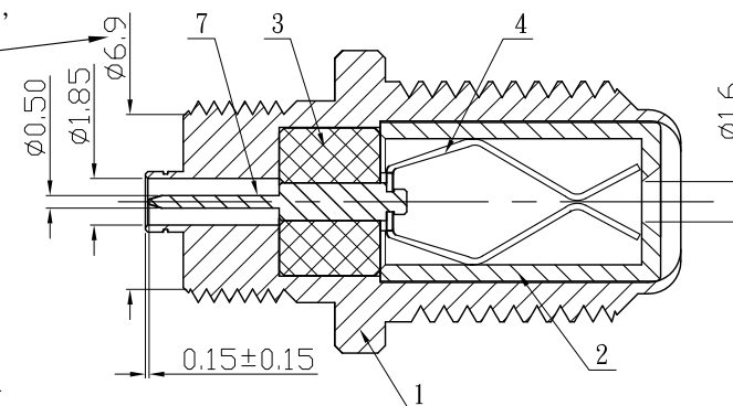
A-A' 剖視圖
