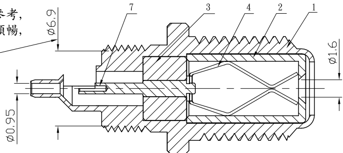
A-A' 剖視圖
