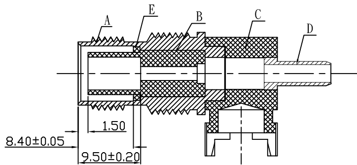
A-A部剖視圖 CD013932001-9
